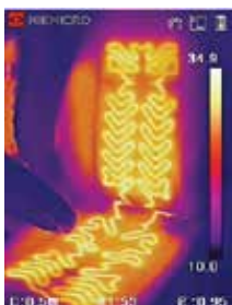
Prikaz grejača sedišta
